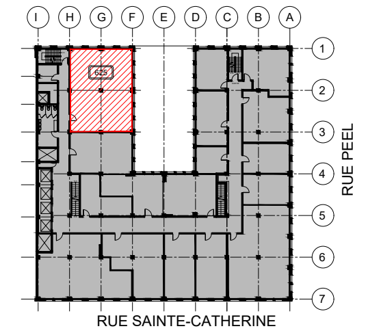
PLAN CLÉ
