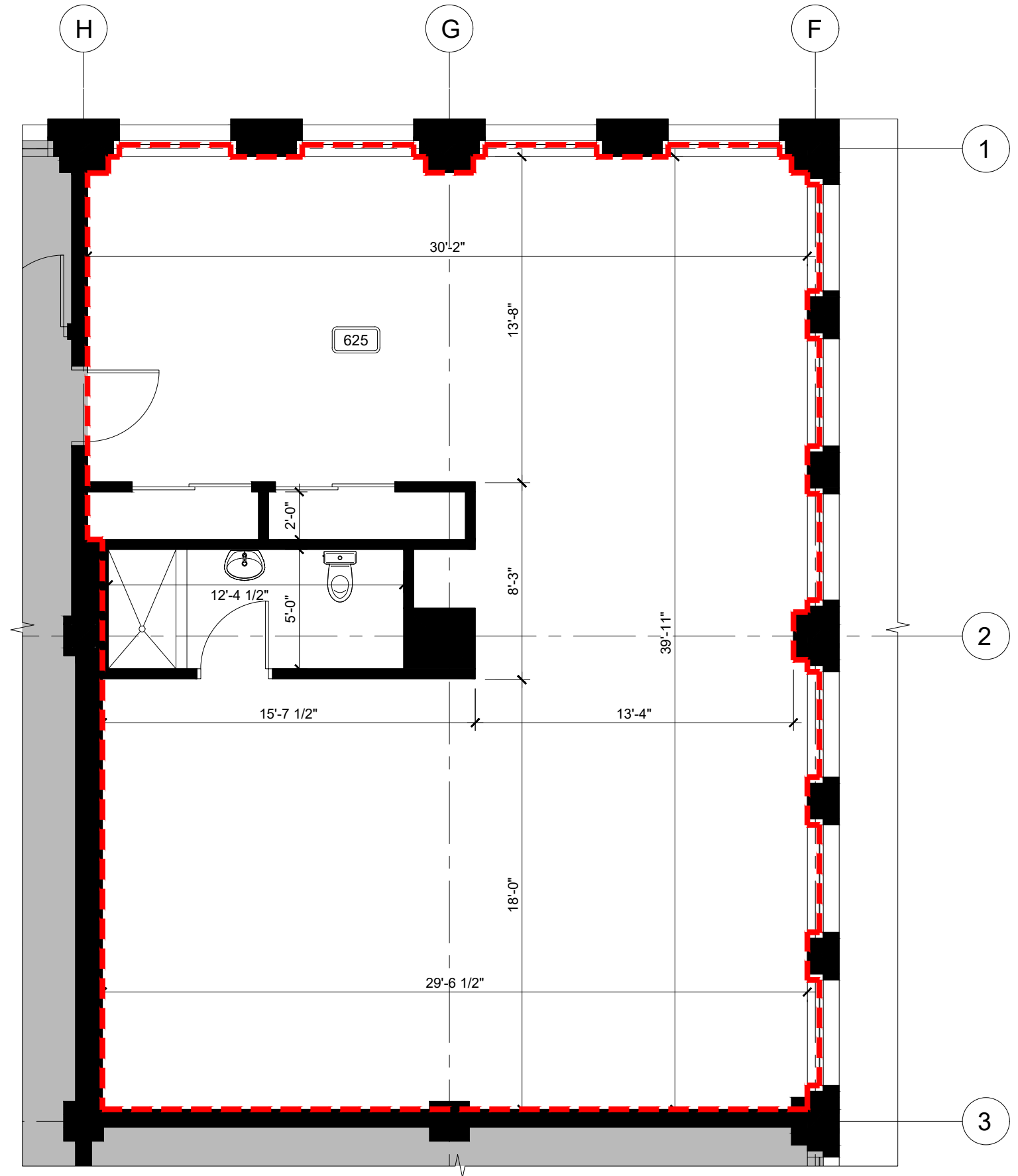
PLAN DE SUITE 625 SCALE / ÉCHELLE: 3/16" = 1'-0"
