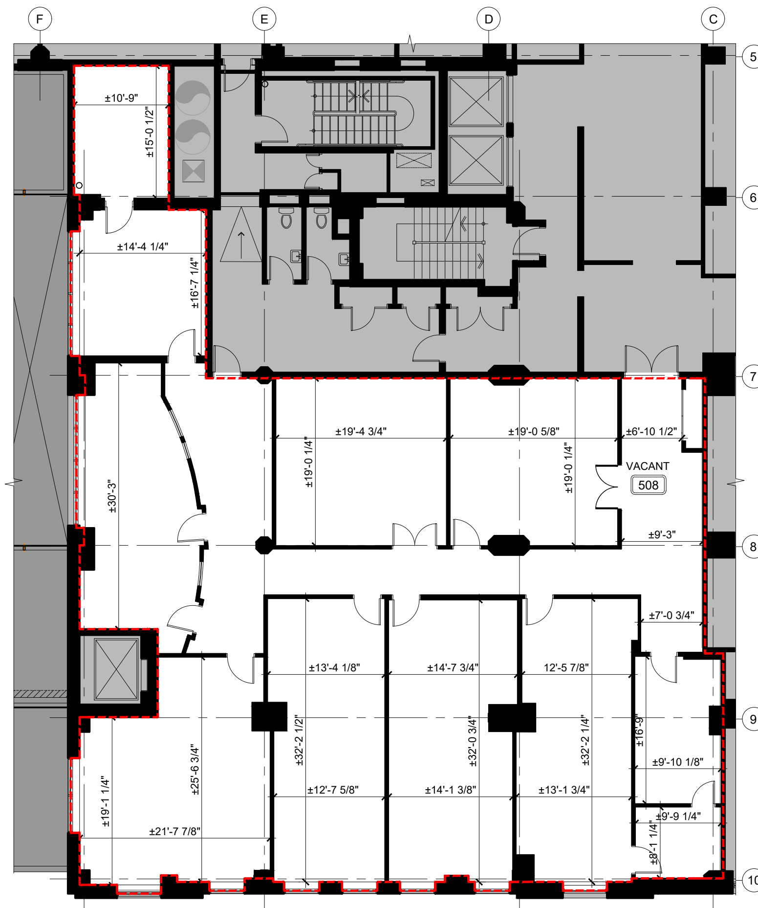
PLAN DE SUITE 508 SCALE / ÉCHELLE: 3/32" = 1'-0"
