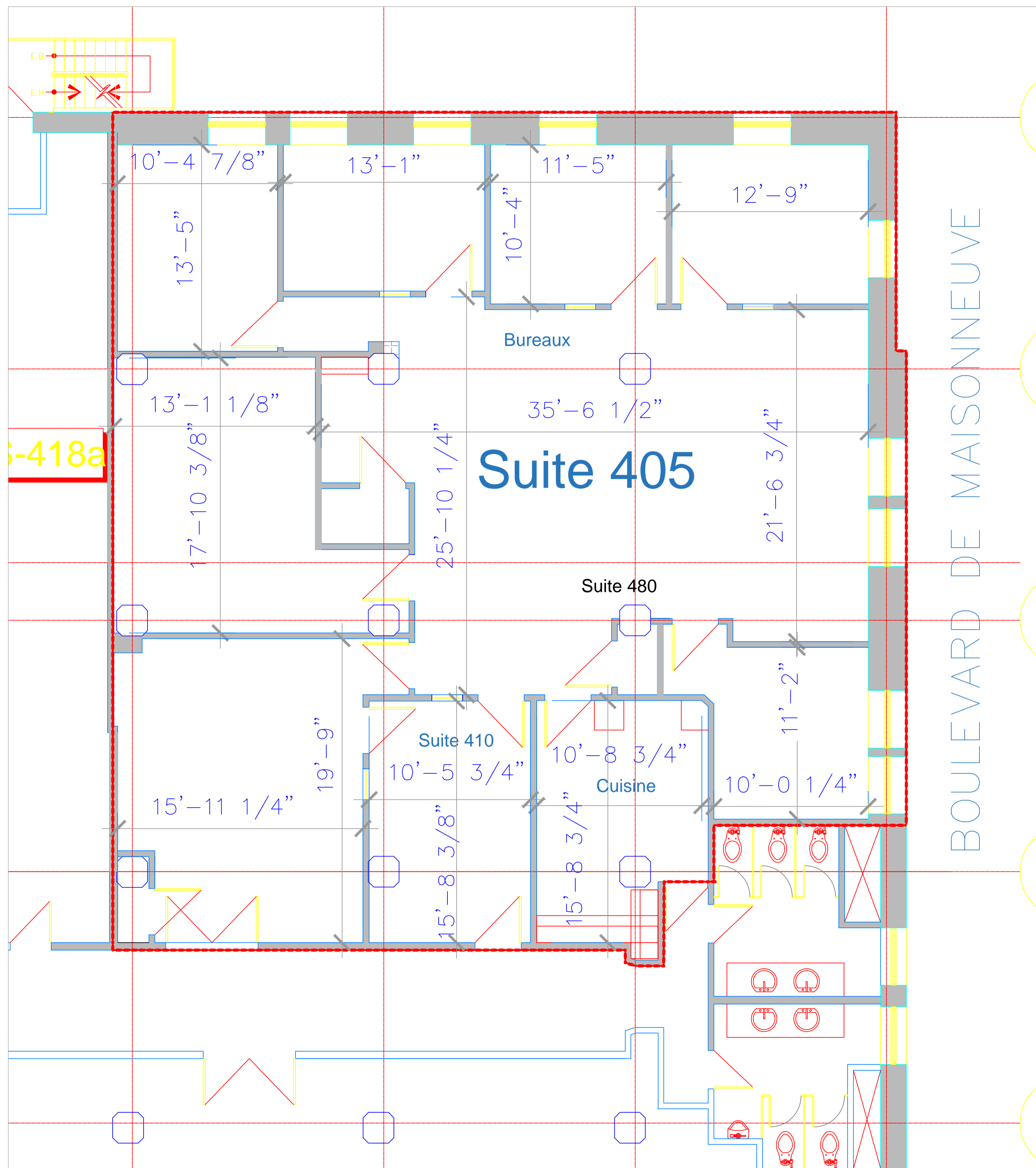
Echele Scale: 6"=1'-0"
