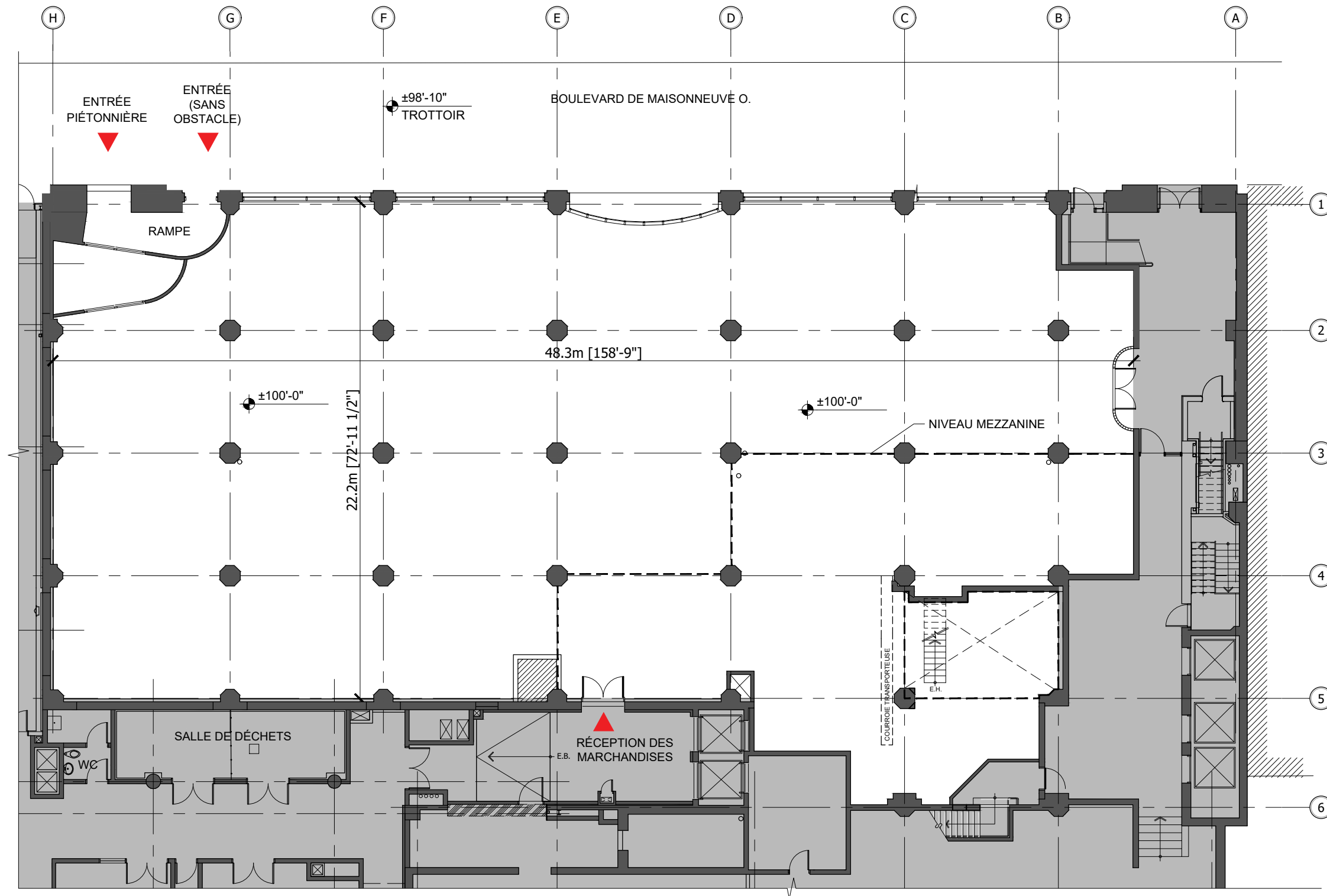
PLAN DU LOCAL - NIVEAU RDC
