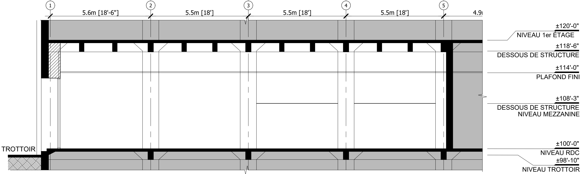
COUPE TRANSVERSALE ÉCHELLE/ SCALE: 1:100
