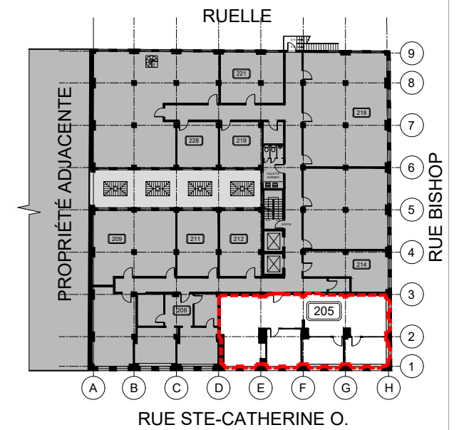
PLAN CLÉ
