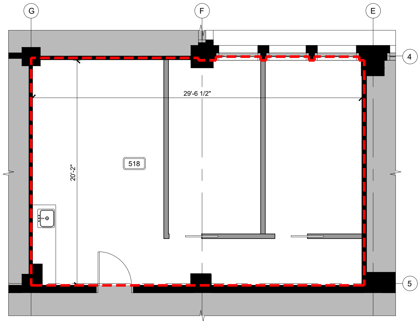
PLAN DE SUITE 518
