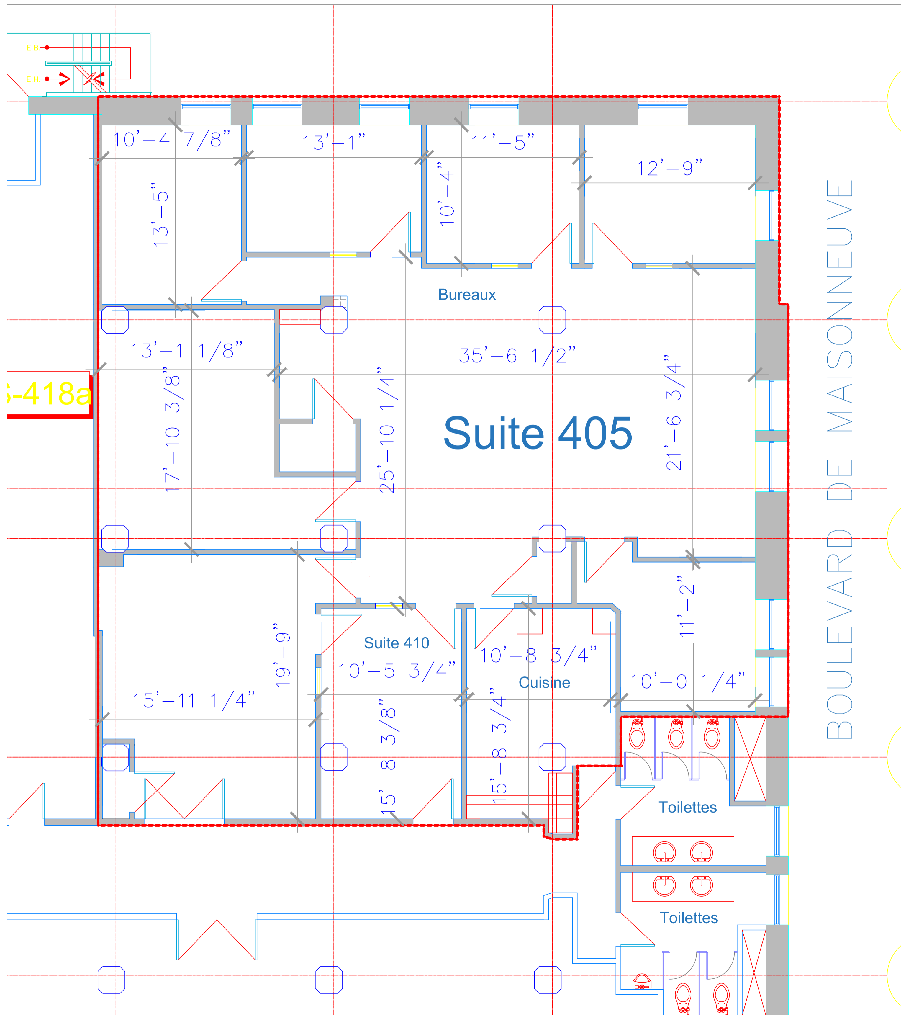
Echele Scale: 6"=1'-0"
